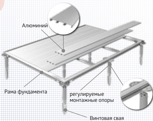
Рис. Свайно винтовой фундамент
